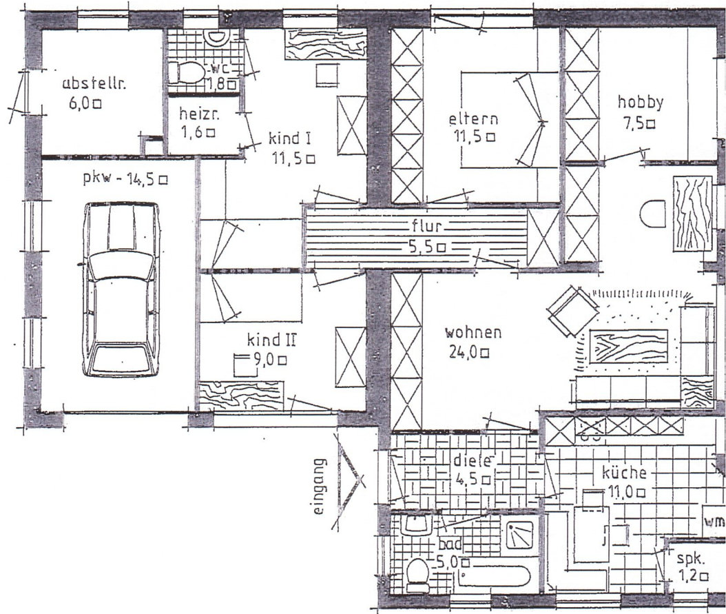
wohnung I (erdgeschoß)
